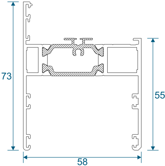
AW607 - Deep Ovolo
